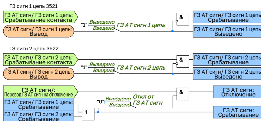
Рисунок 2.12 – Функциональная схема логики сигнальной ступени ГЗ АТ
