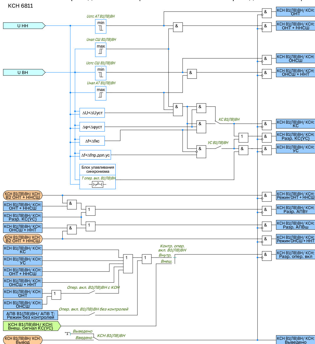
Рисунок 2.27 – Функциональная схема КСН В1(ЛВ) ВН
